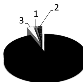
controle (n=90)
